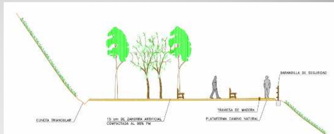
Secció transversal de l'Àrea de descans Can salgado
