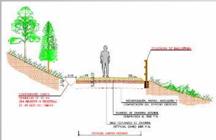
Secció transversal del Camí Natural
